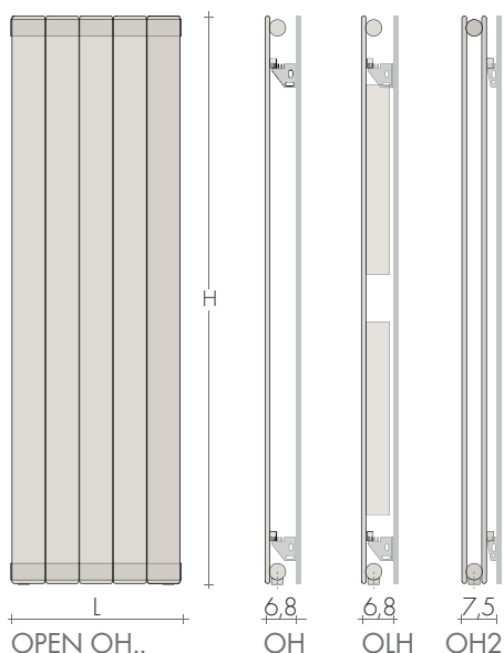
OH Panneau vertical et collecteurs horizontaux
