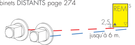
RACCORDS DISTANTS Art. REM 42,10€ Entraxe raccord à l'arrière du radiateur: ▲▽ L-6 cm Robinets DISTANTS page 274
