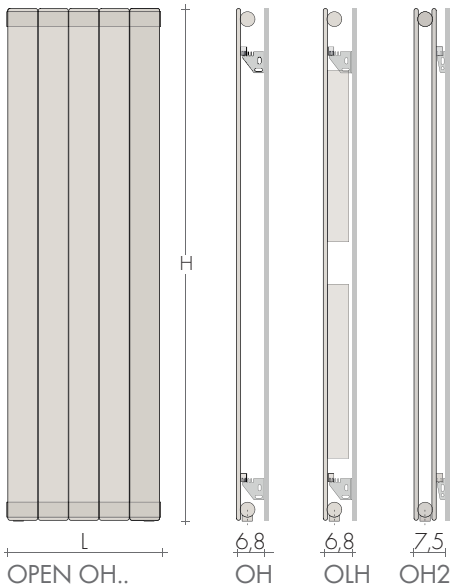
OH Panneau vertical et collecteurs horizontaux
