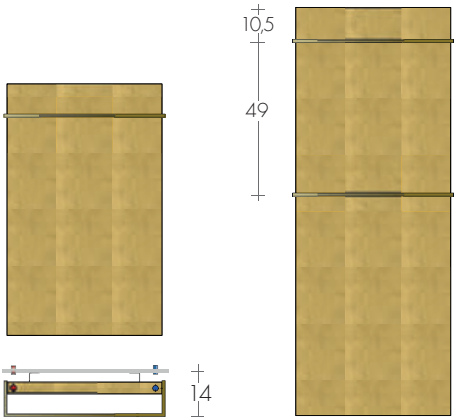
PLATT FO/FA 80-49 PLATT FO/FA 84-50 PLATT FO/FA 130-50 133-50 / 140-60
