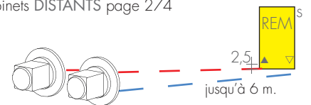
RACCORD DISTANTS Art. REM 42,10€ Entraxe raccord à l'arrière du radiateur: ▲▽ L - 5 cm Robinets DISTANTS page 274
