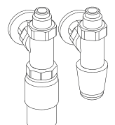
Es. Valvola termostatica non sporgente
