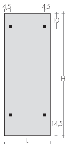
FISSAGGI Mensole G30 comprese
