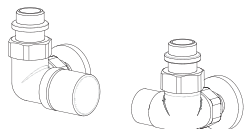
KIT VALVOLE CYL termostaticabile con comando LATERALE, pag.273
