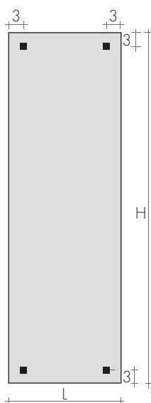
FISSAGGI Mensole comprese
