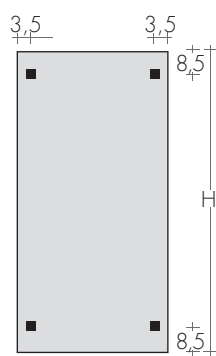
FISSAGGI Mensole Art. G30 comprese
