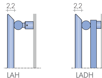
Bordi superiore e laterali delle piastre LAMINA
