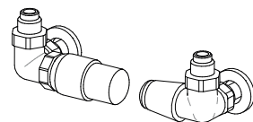
KIT ROBINETS TON commande LATERALE, avec tête thermostatique, p. 269
