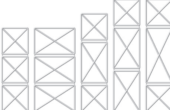
RAW3 157-50 RAW3 157-77 RAW3 183-50 RAW3 210-50A RAW3 210-50B RAW3 250-60
