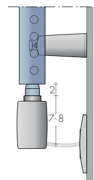
Art. R...IIF, avec Faston pour Thermostat Intégré
