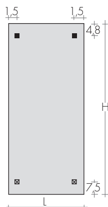
FISSAGGI Mensole B70 comprese
