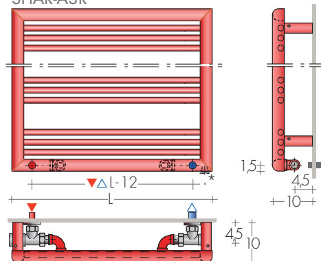
SHAR-A3R
