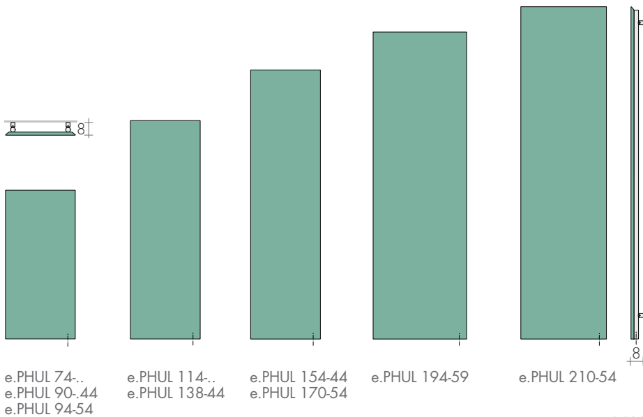
RAM page 277
